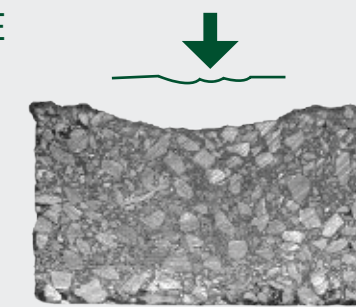
Avec seulement 0.8% de SELENIZZA® après 30 000 cycles
